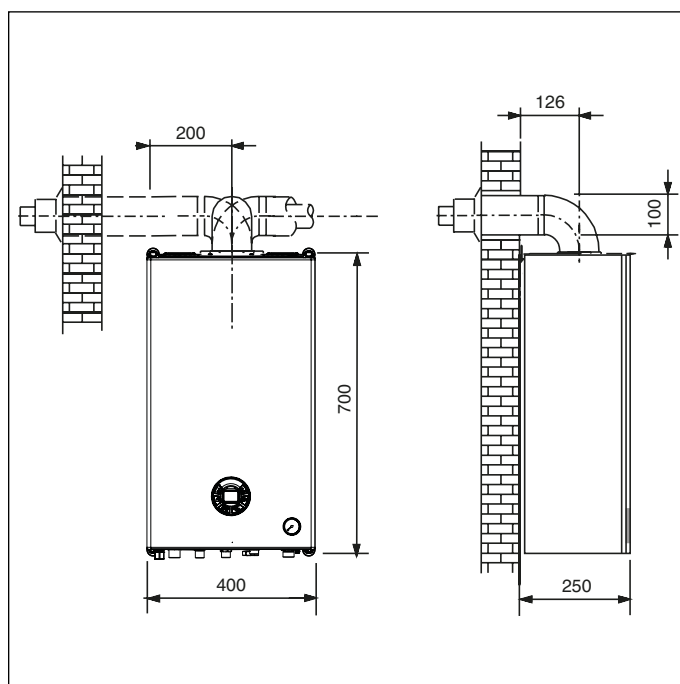
Obr. 14 Velikosti koaxiálního potrubí typ C13 - C33
