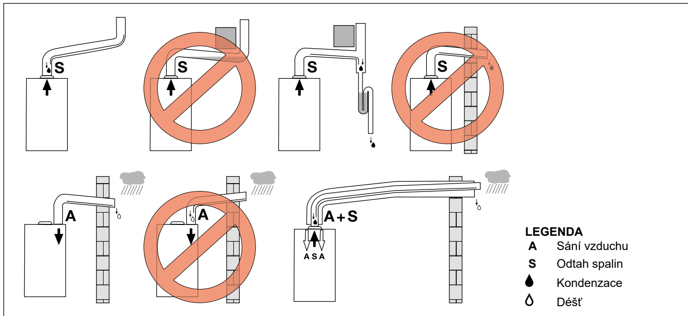
Obr. 8 Příklady instalace
