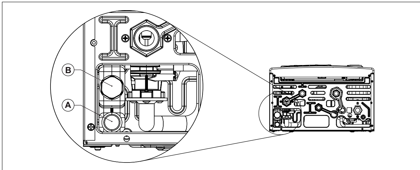
Obr. 20 Vypuštění kondenzátu
