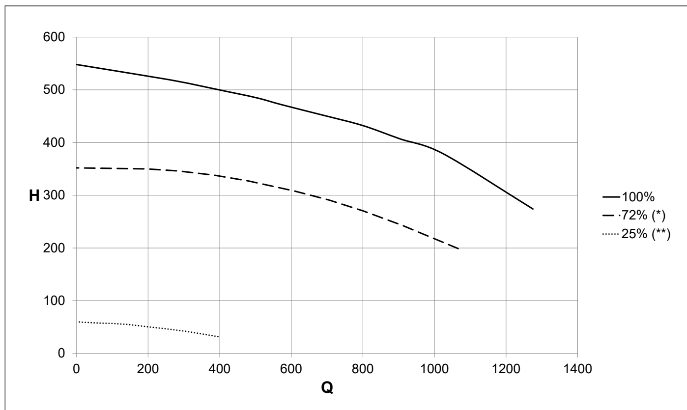
Obr. 22 Dostupná hlava
