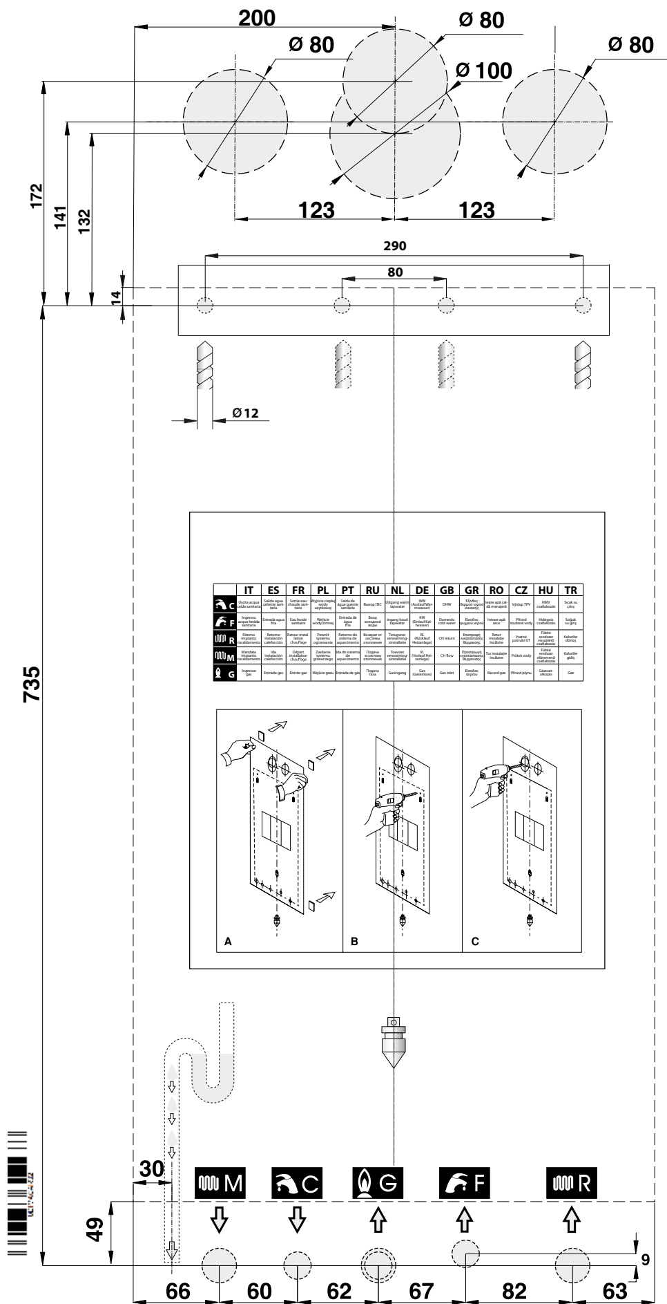
Obr. 5 Papírová šablona
