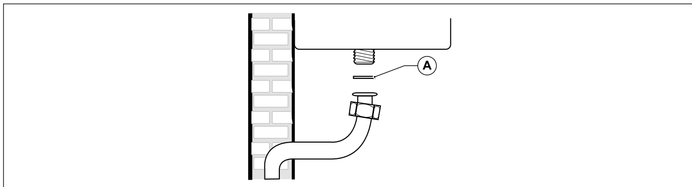
Obr. 19 Připojení k rozvodu plynu
