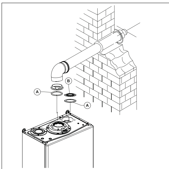
Obr. 13 Koaxiální potrubí typu C13 - C33
