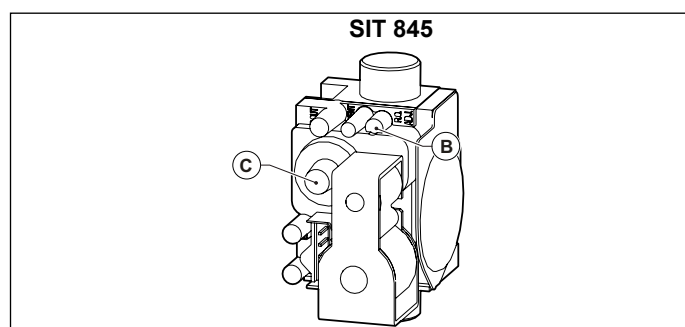
Obr. 25 Nastavení plynového ventilu
