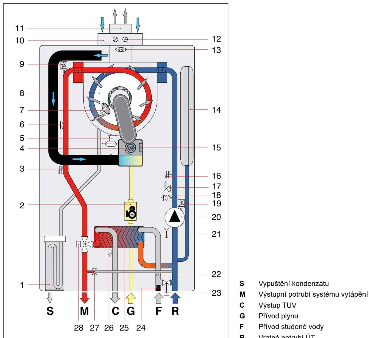
Obr. 4 Uspořádání kotle
