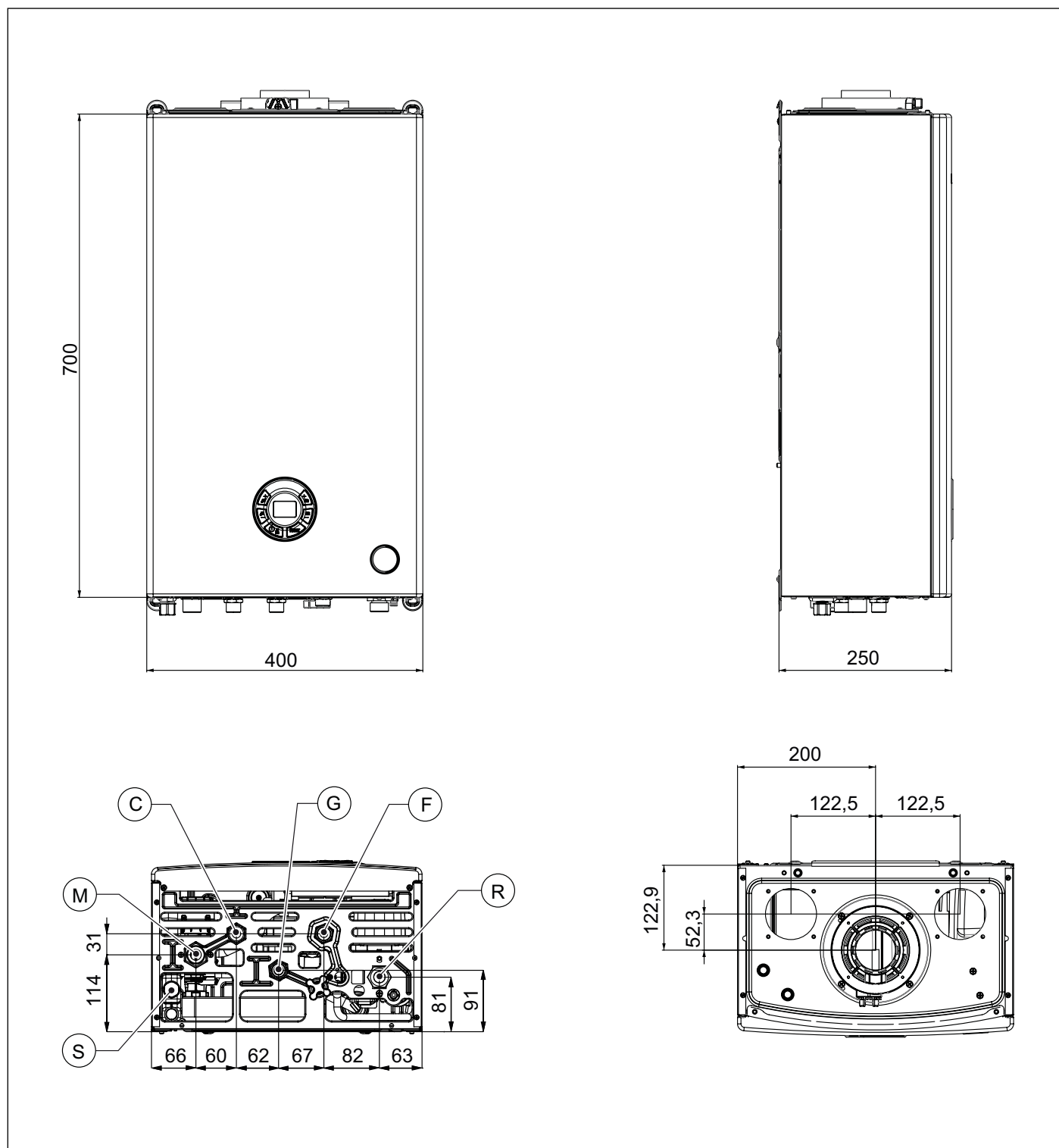
Obr. 3 Rozměry
