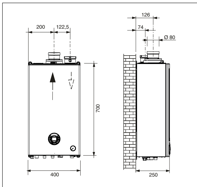
Obr. 16 Rozměry pro dělené potrubí
