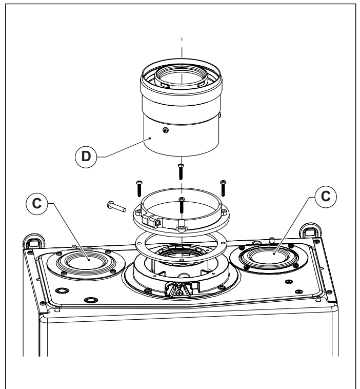
Obr. 7 Instalace koaxiální sady
