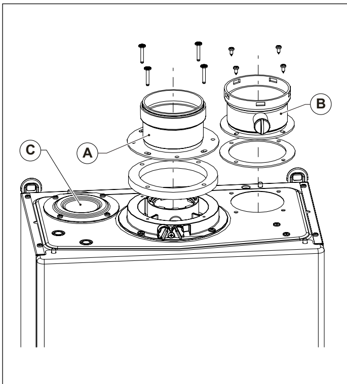
Obr. 6 Instalace sady pro samostatná potrubí
