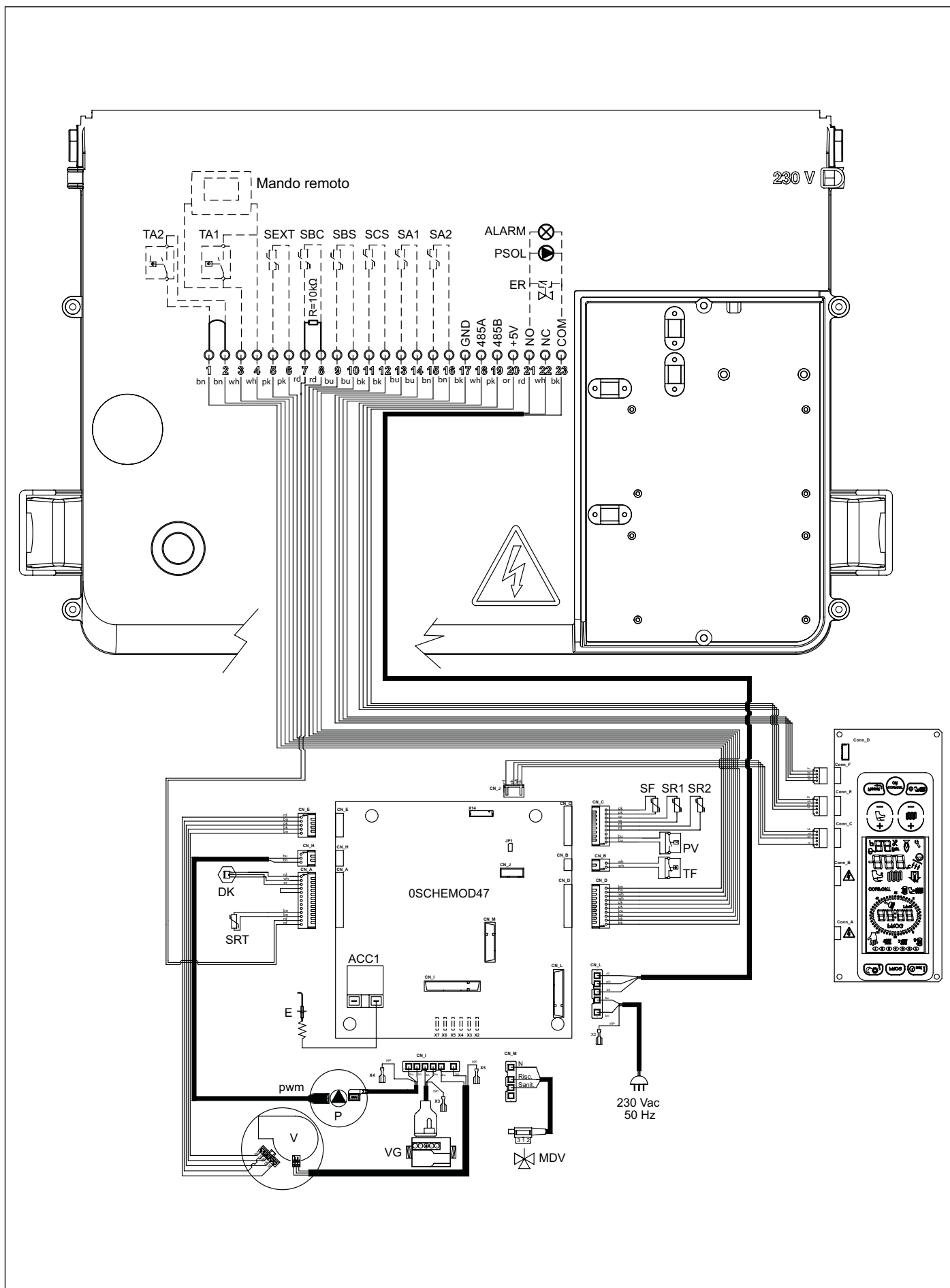
Fig. 32 Esquema eléctrico KRB
