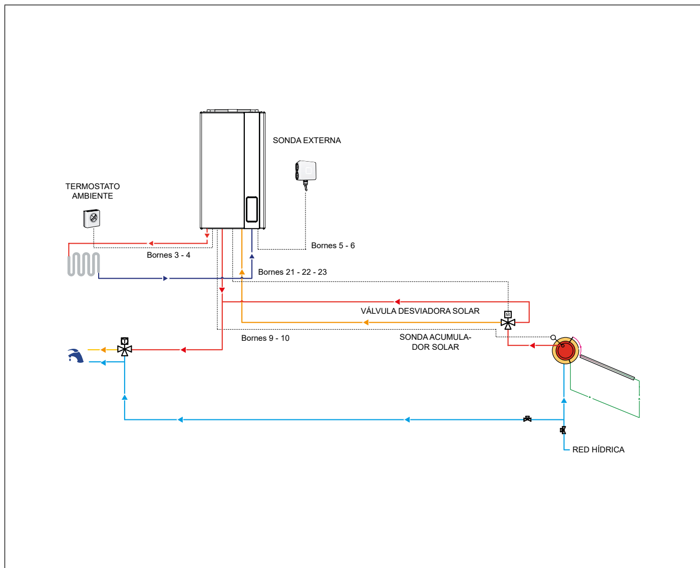
Fig. 27 Esquema de conexión sistema solar a circulación natural con caldera combinada
