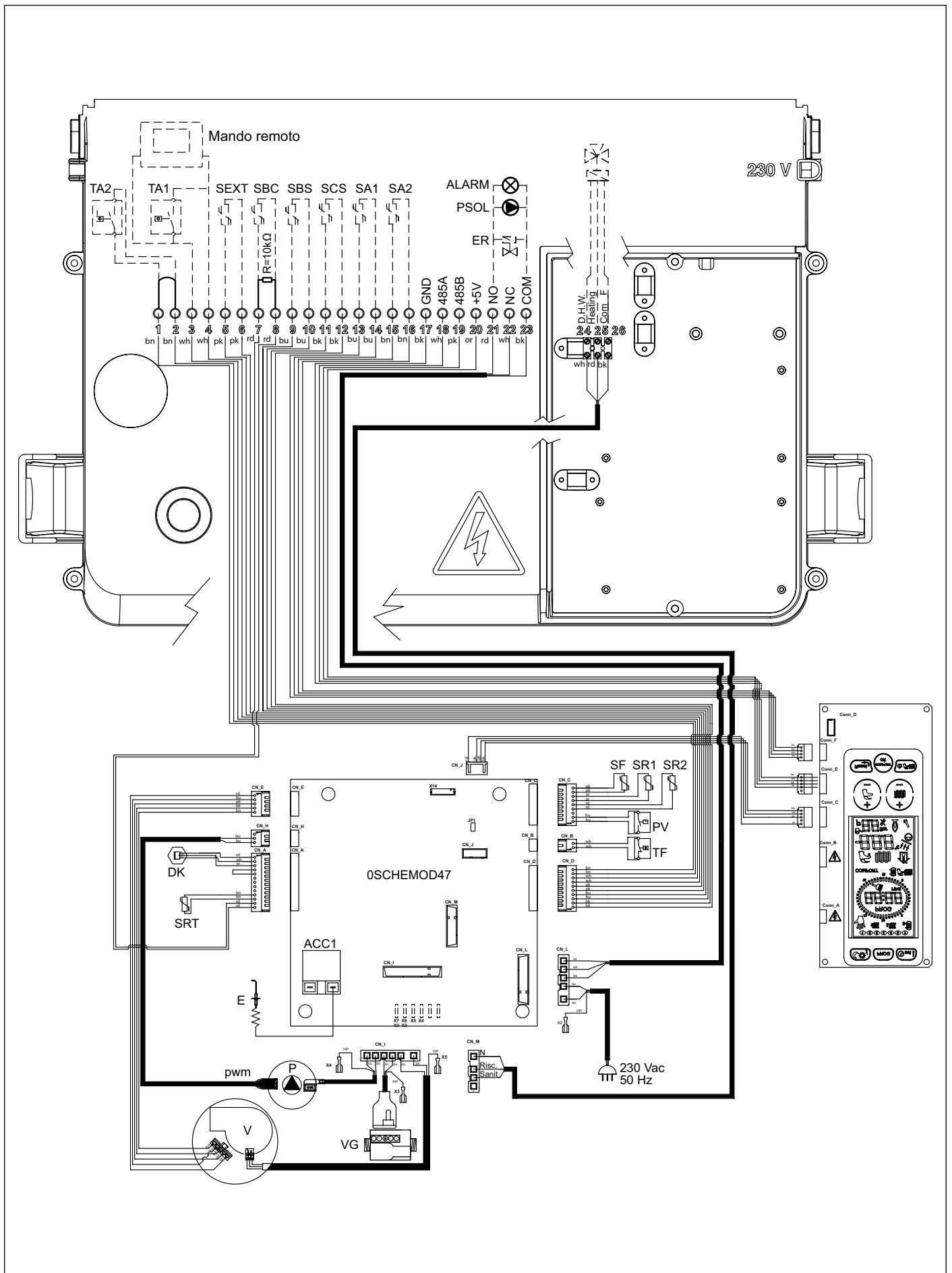
Fig. 29 Esquema eléctrico KR
