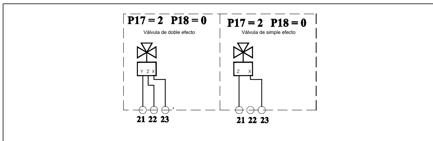
Fig. 28 Esquema de conexión relé multifunción (X= neutro; Y= en caldera; Z= al colector)
