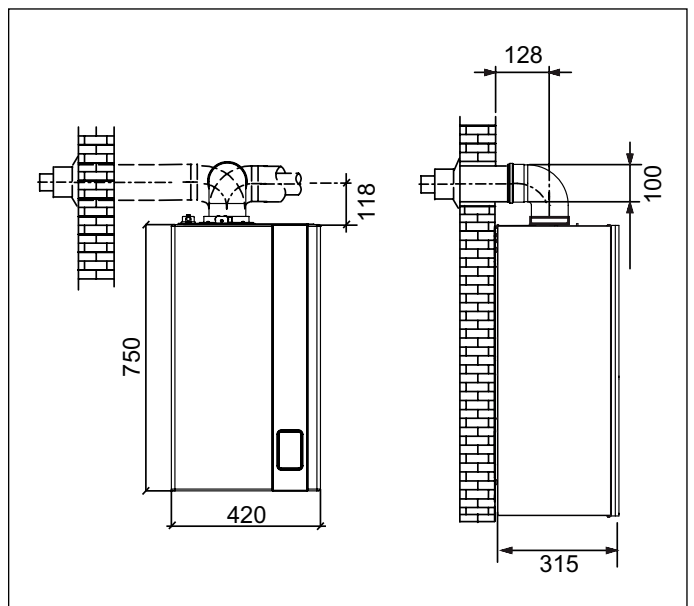
Fig. 12 Distancias conductos coaxiales tipo C33
