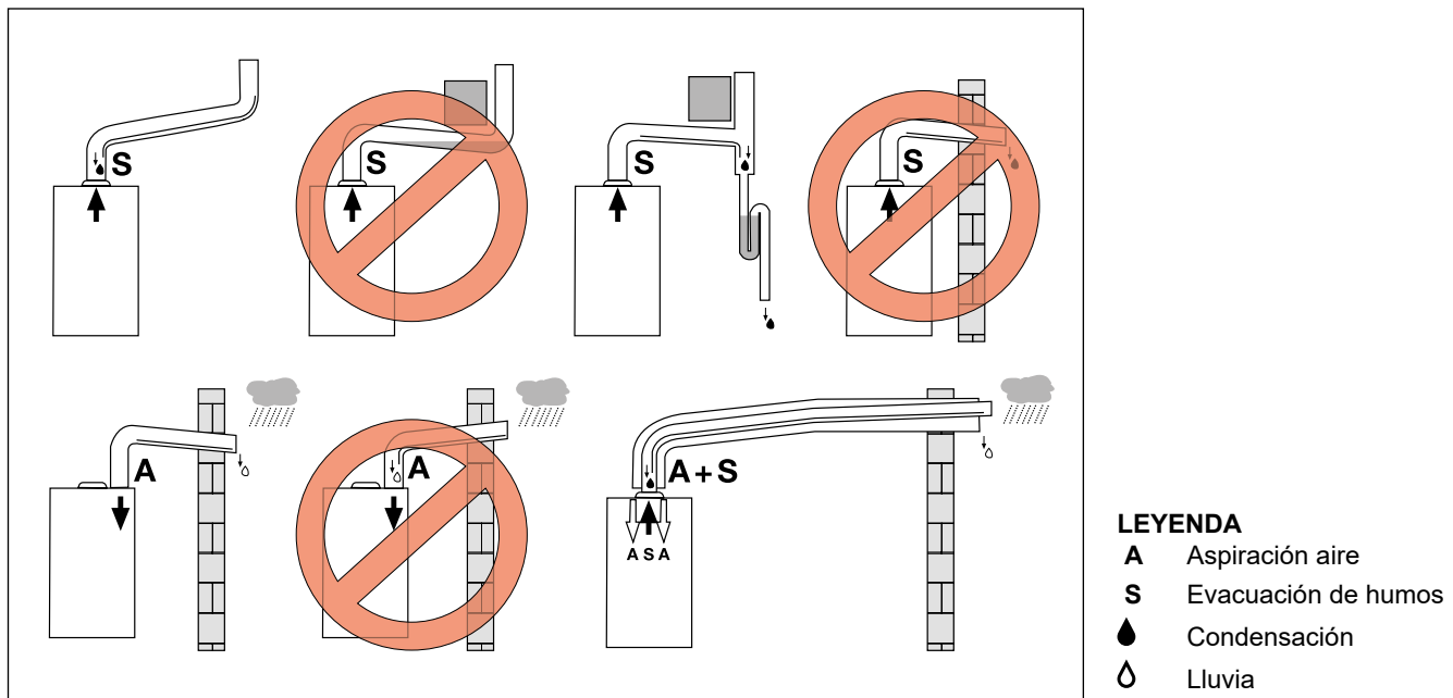
Fig. 10 Ejemplos de instalación
