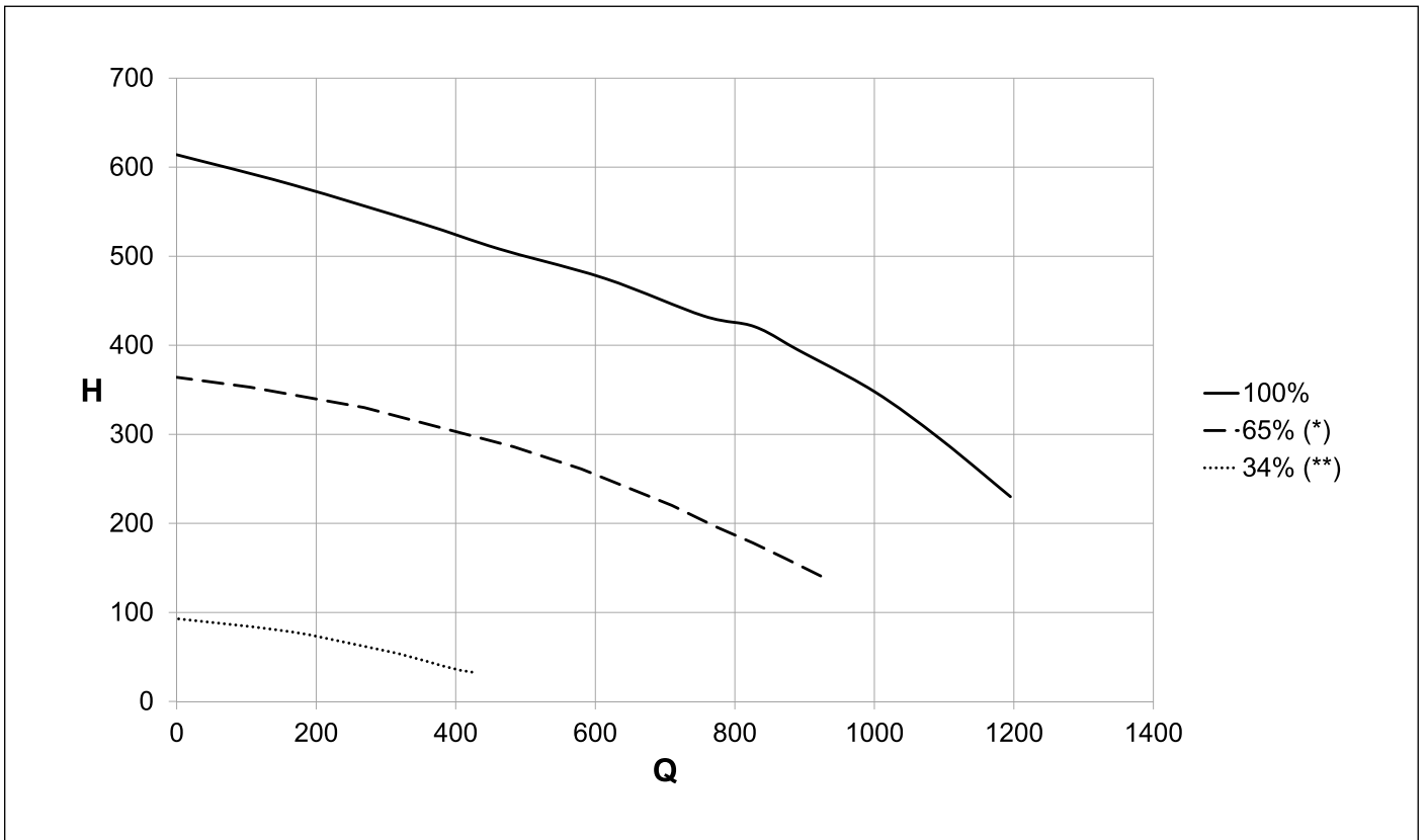
Fig. 22 Alturas residuales disponibles KC-KR-KRB 28
