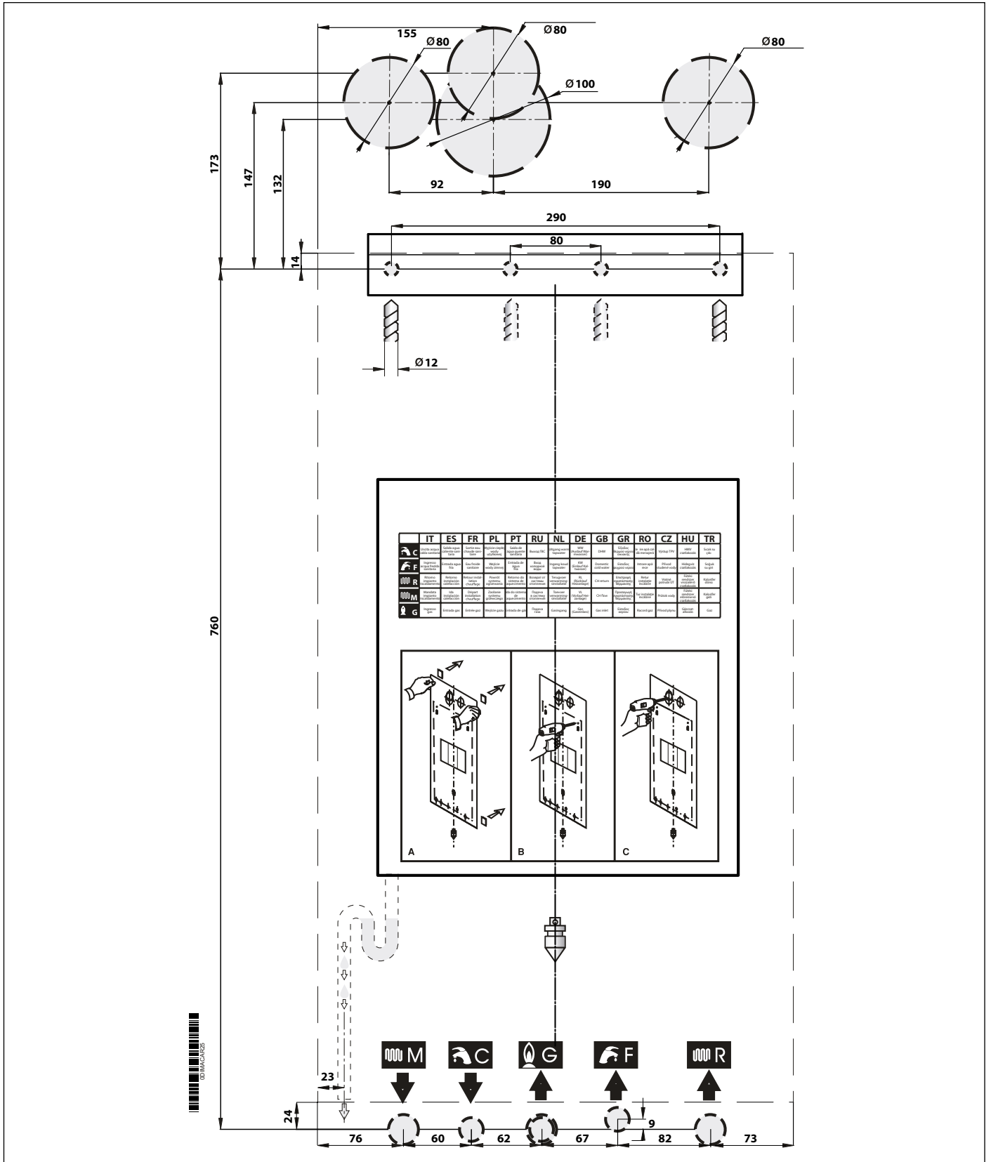
Fig. 9 Plantilla de instalación
