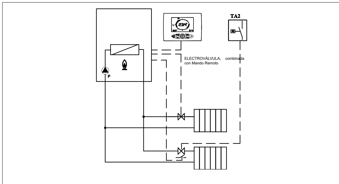
Fig. 33 Relé con mando a distancia y TA2
