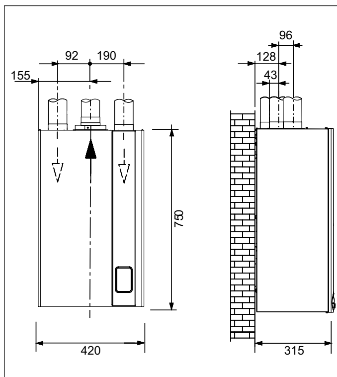
Fig. 14 Dimensiones conductos coaxiales tipo C43 - C53 - C83
