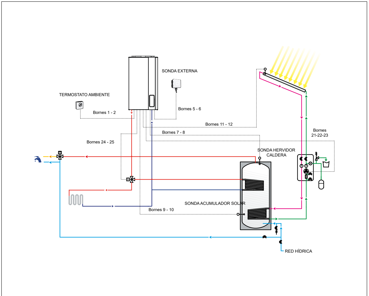
Fig. 30 Esquema de conexión sistema solar a circulación forzada con caldera sólo calefacción
