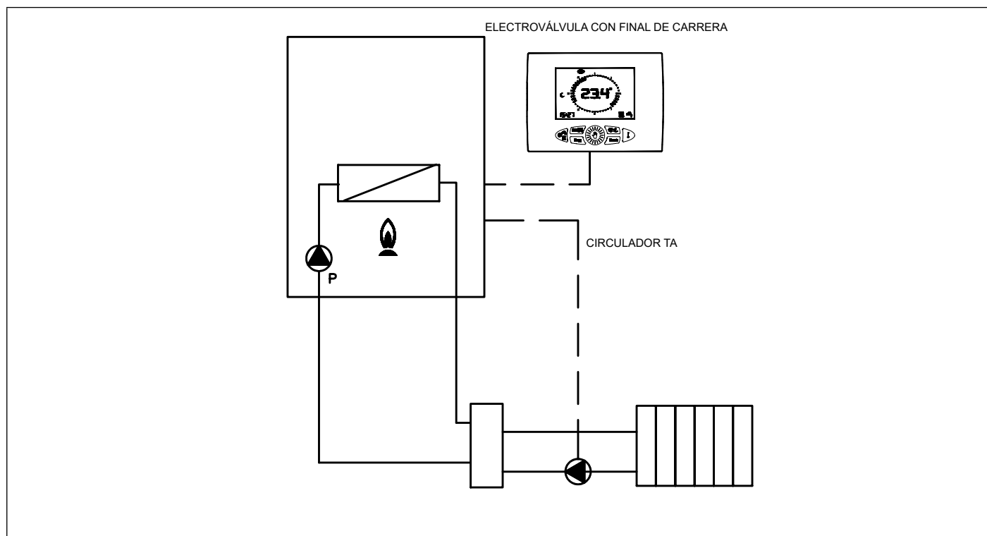
Fig. 34 Relé con pedido a distancia (P17=1)
