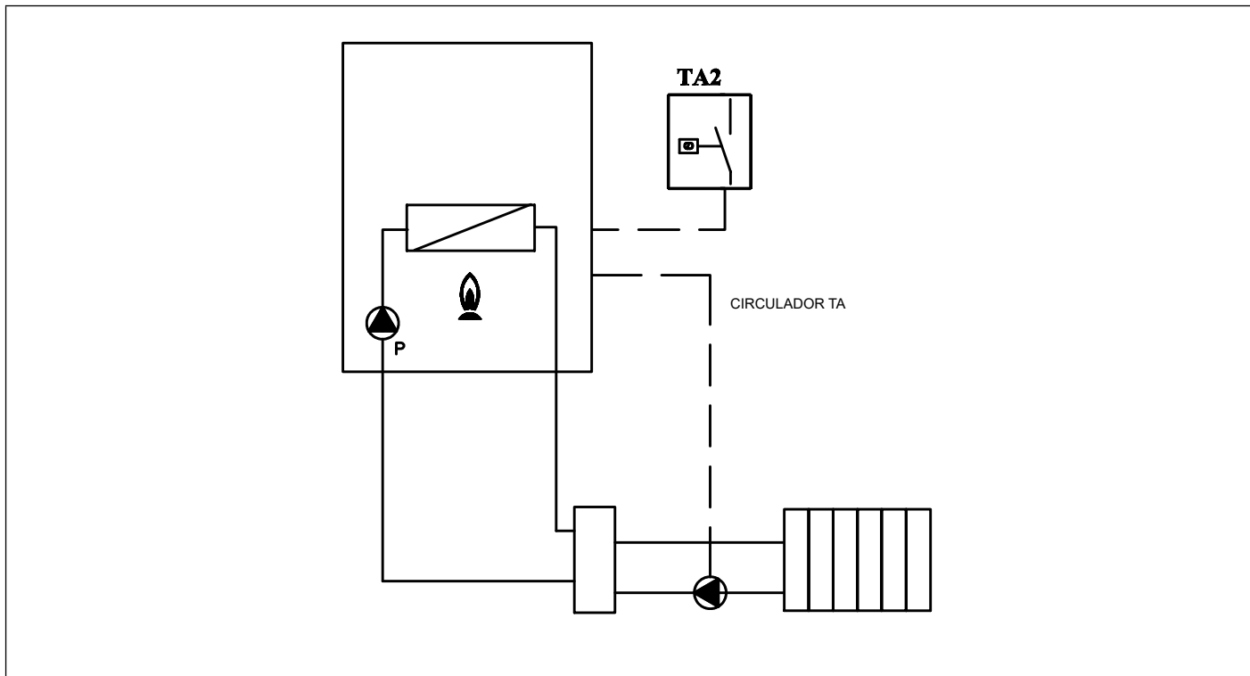
Fig. 35 Relé con pedido (P17=3)
