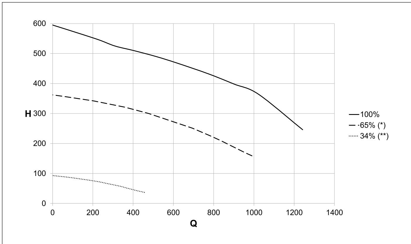
Fig. 23 Alturas residuales disponibles KC-KR-KRB 32
