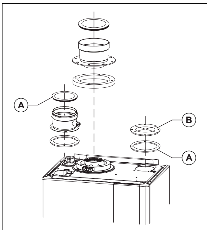
Fig. 13 Conductos coaxiales tipo C43 - C53 - C83
