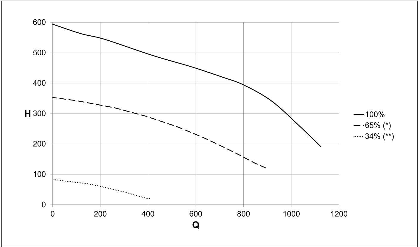
Fig. 21 Alturas residuales disponibles KC-KR-KRB 24
