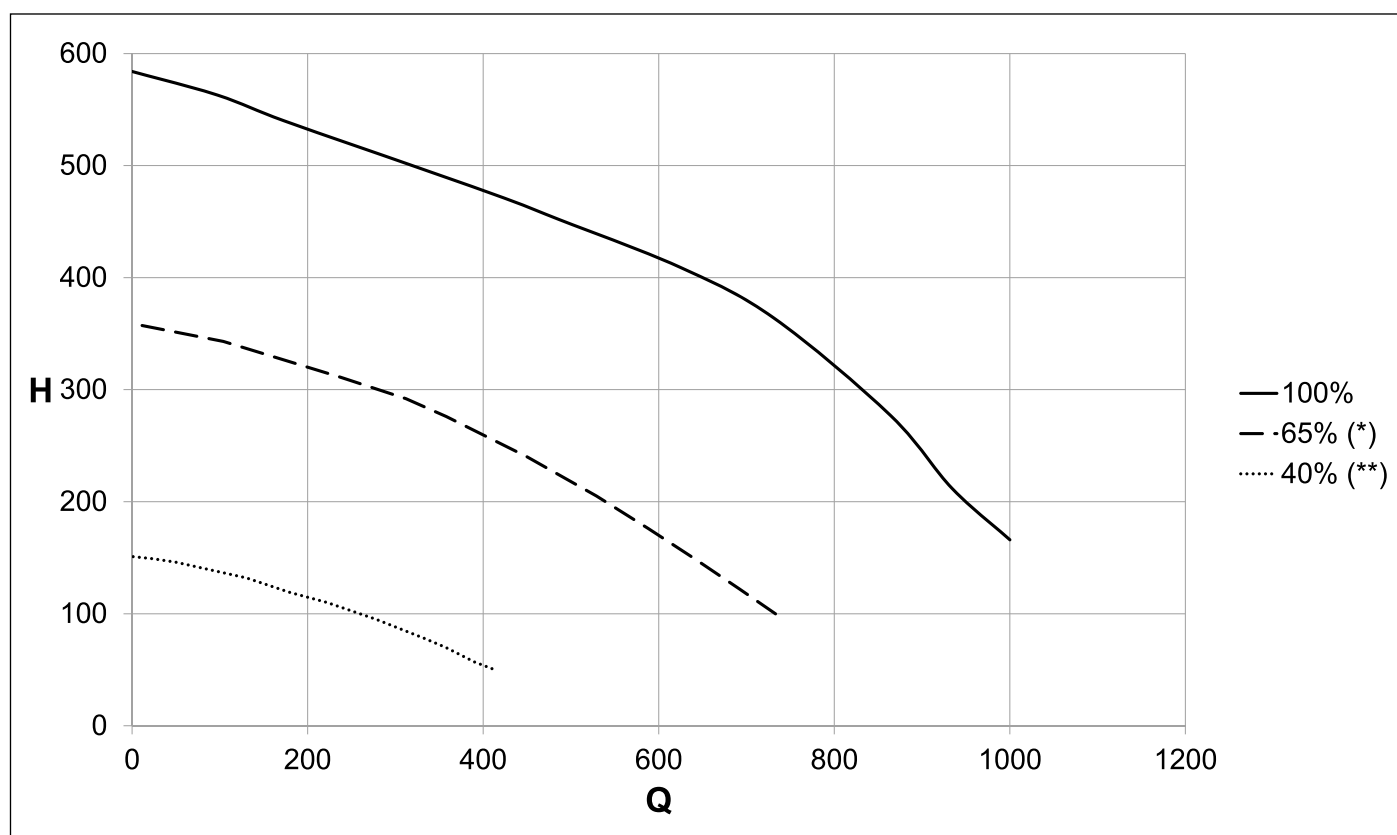
Fig. 20 Alturas residuales disponibles KC-KR-KRB 12
