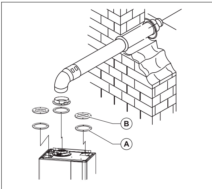
Fig. 11 Conductos coaxiales tipo C33
