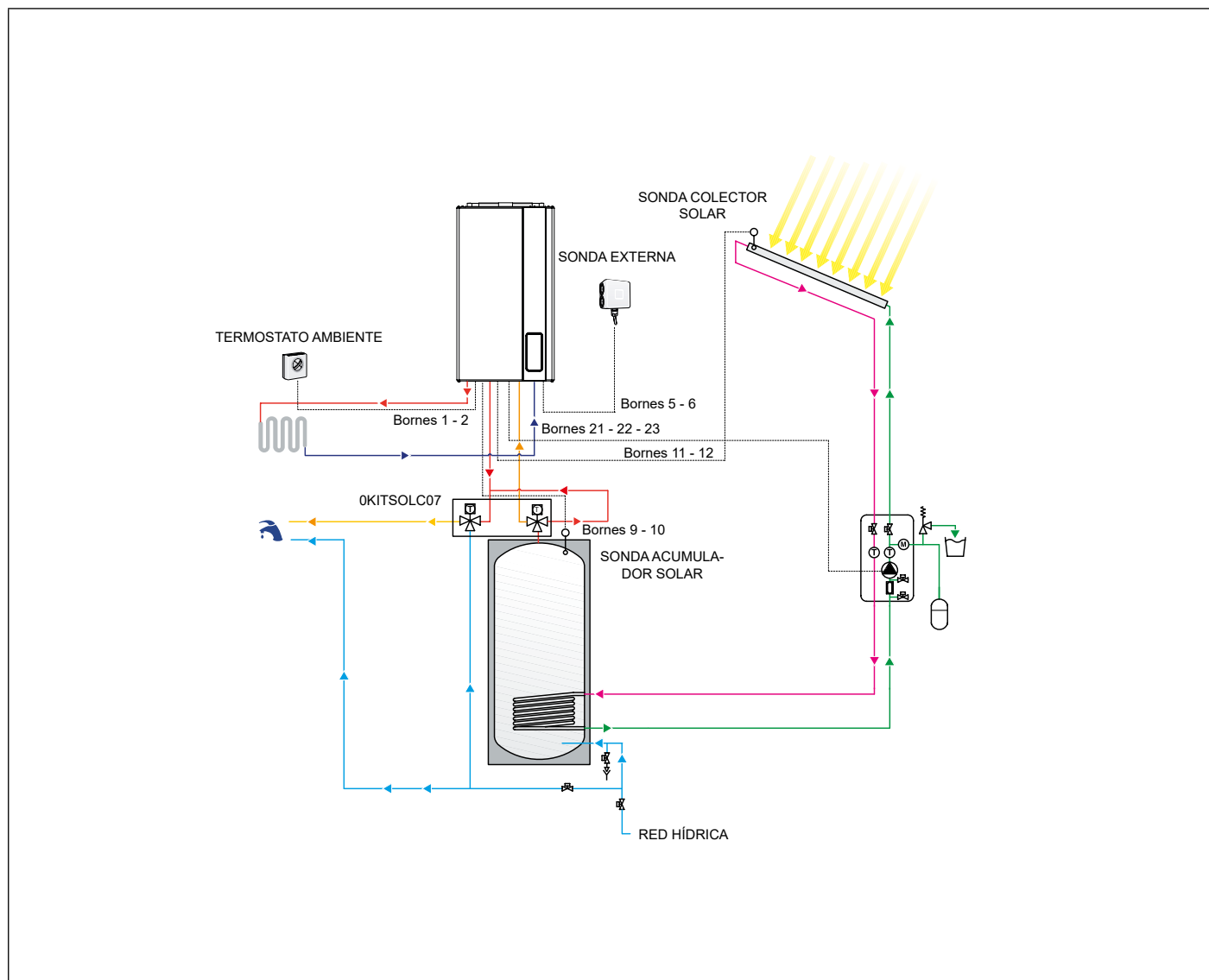
Fig. 25 Esquema de conexión sistema solar a circulación forzada con caldera combinada
