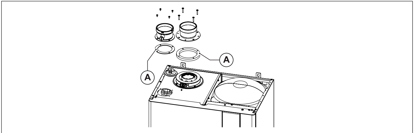
Fig. 11 Conductos desdoblados tipo tipo C43 - C53 - C83
