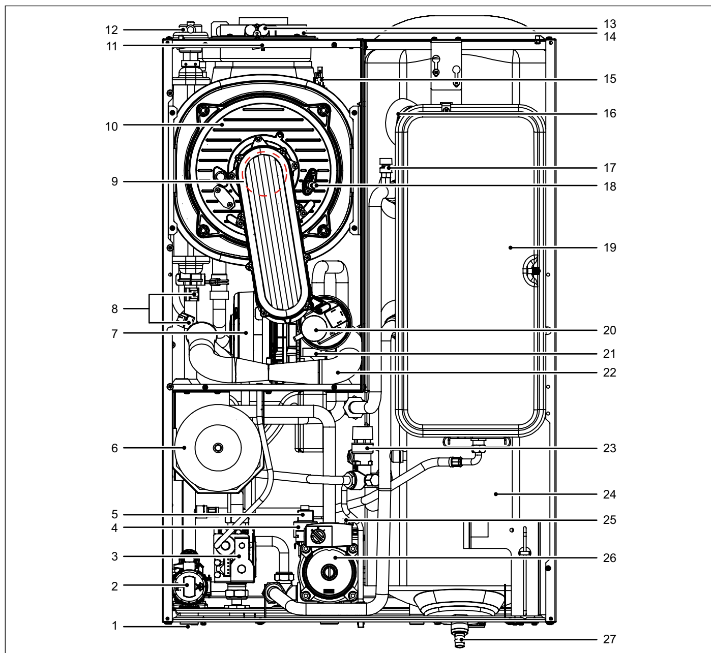
Fig. 4 Componentes principales
