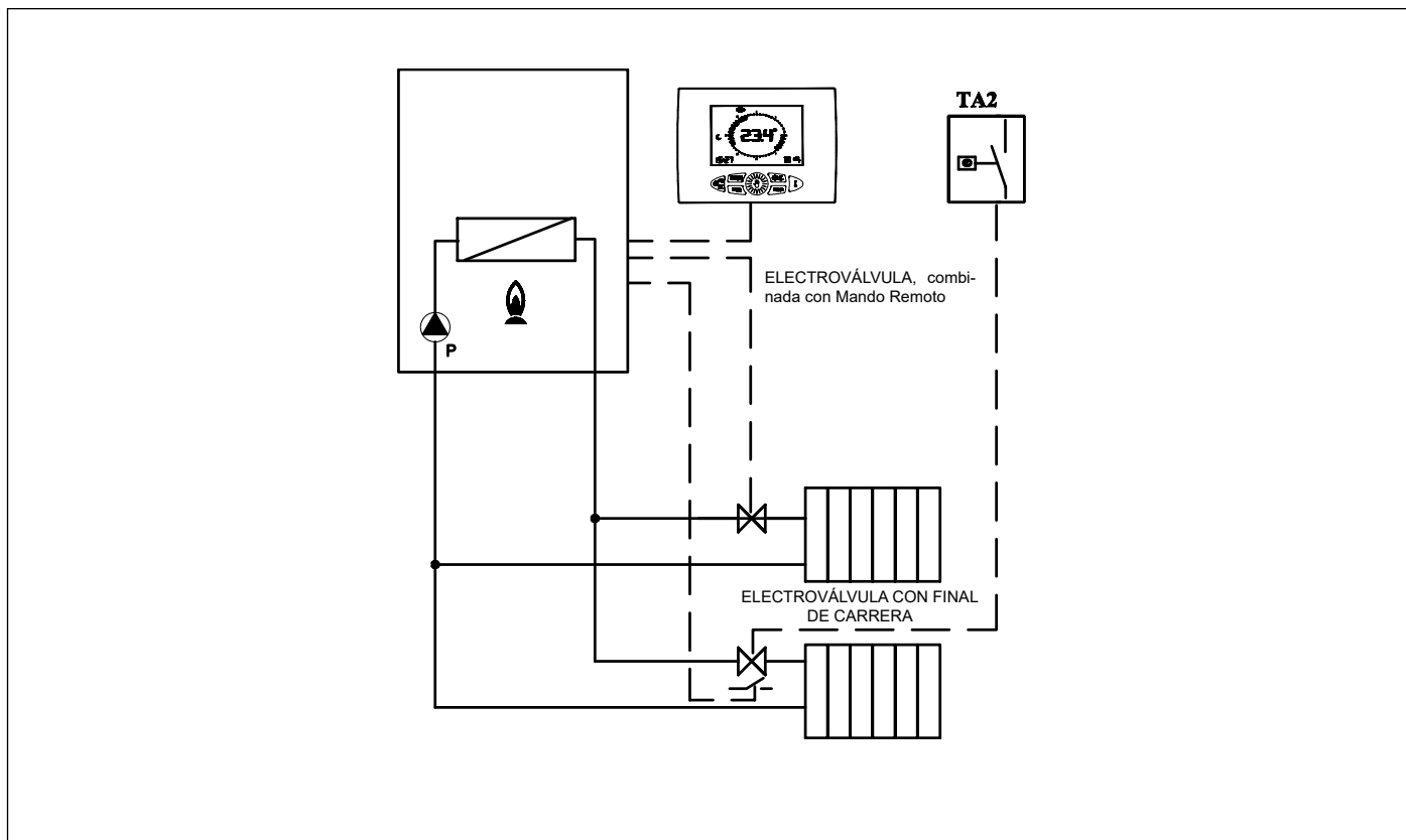
Fig. 21 Relé con mando a distancia y TA2
