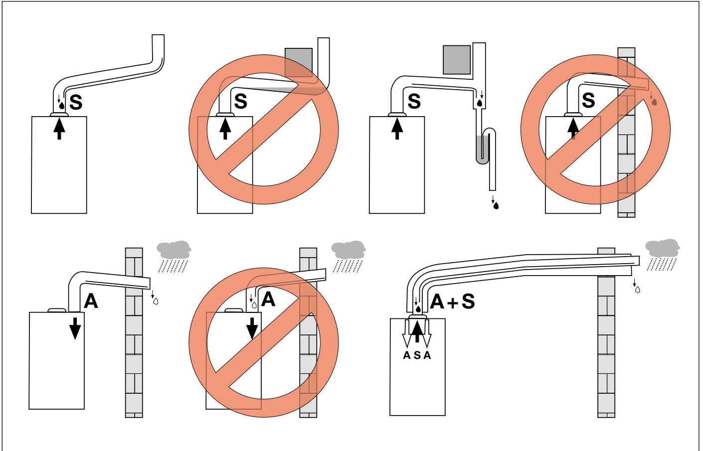
Fig. 8 Ejemplos de instalación
