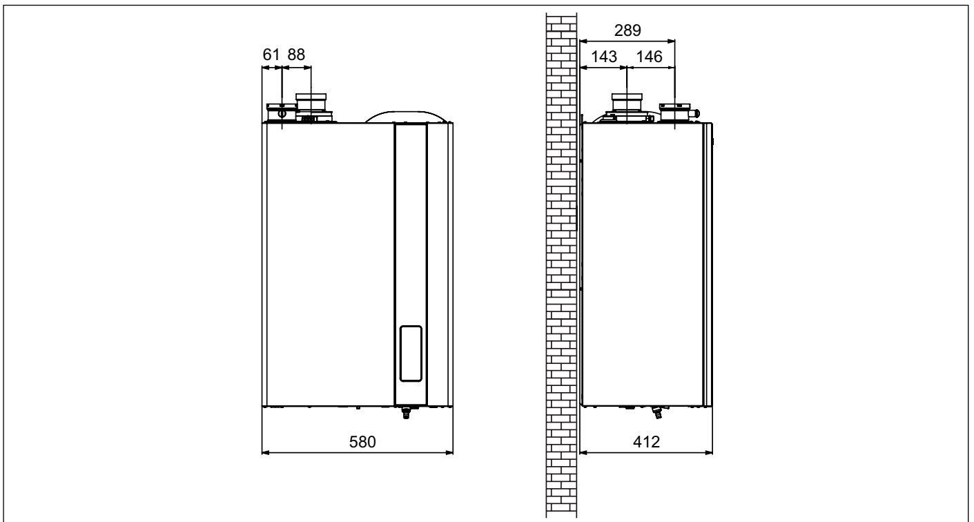
Fig. 12 Dimensiones conductos desdoblados tipo C43 - C53 - C83
