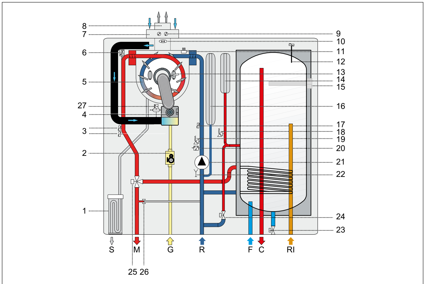
Fig. 5 Esquema hidráulico
