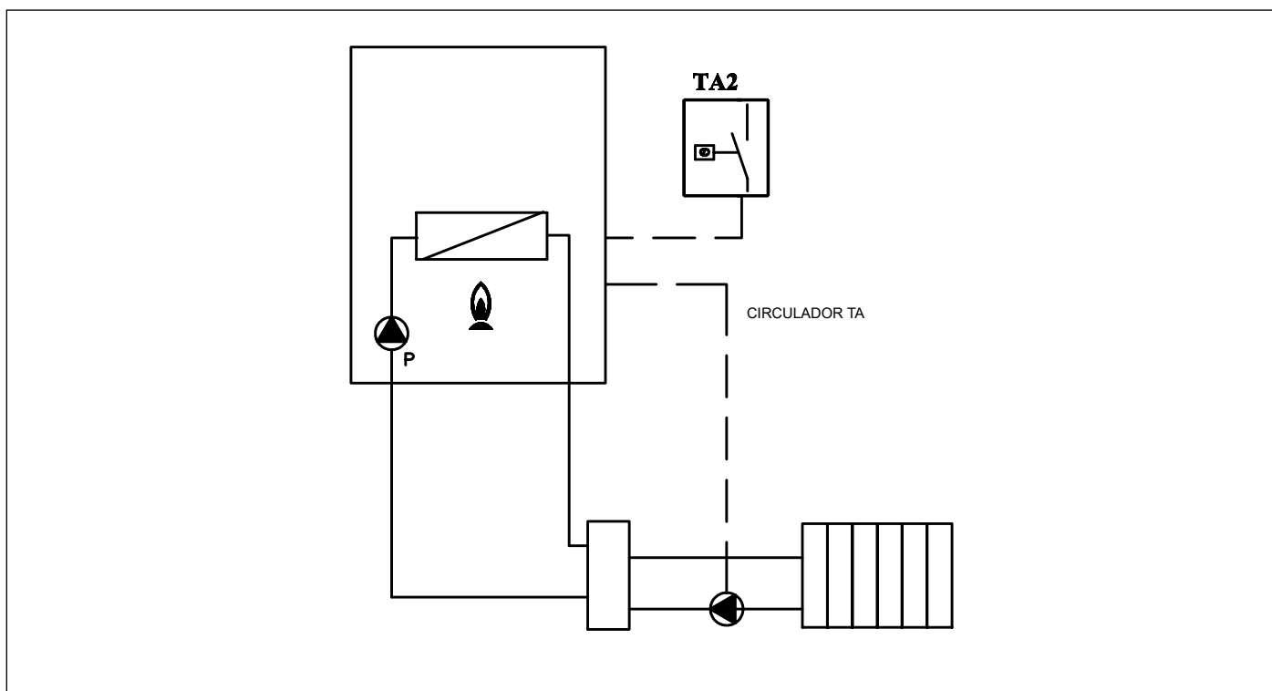
Fig. 24 Relé con pedido (P17=3)
