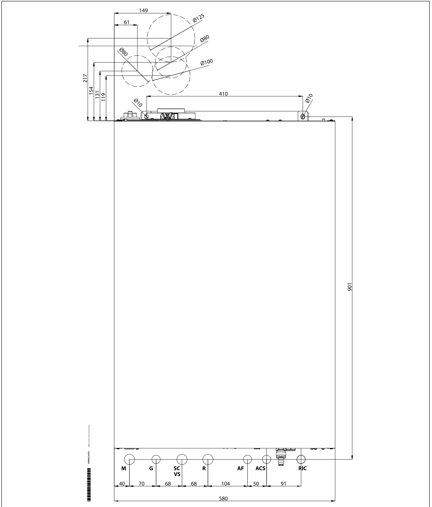
Fig. 6 Plantilla de instalación
