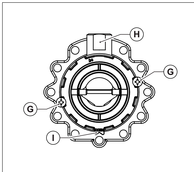
Fig. 29 Orientación de montaje
