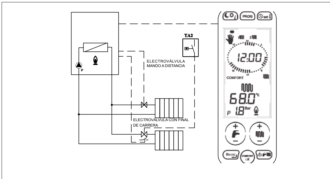
Fig. 22 Relé con programación interfaz y TA2
