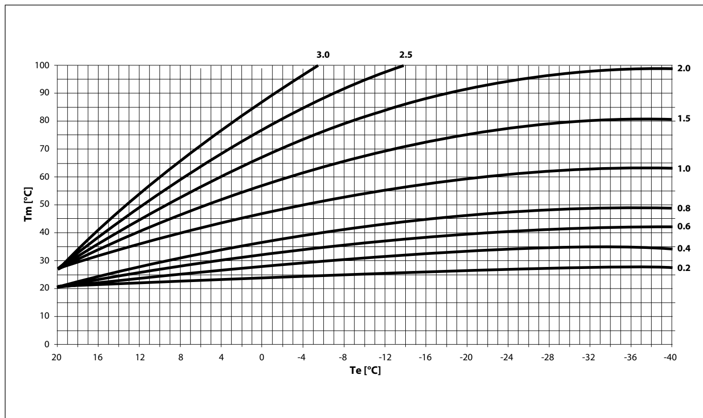
Fig. 16 Curvas de termostatación
