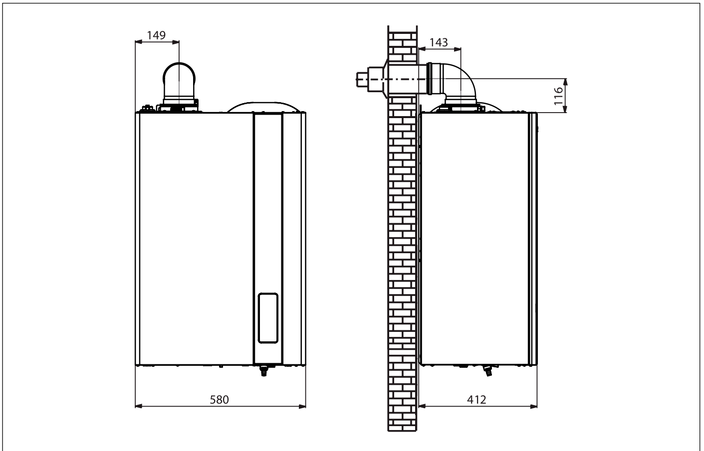
Fig. 10 Dimensiones conductos coaxiales tipo C13 - C33
