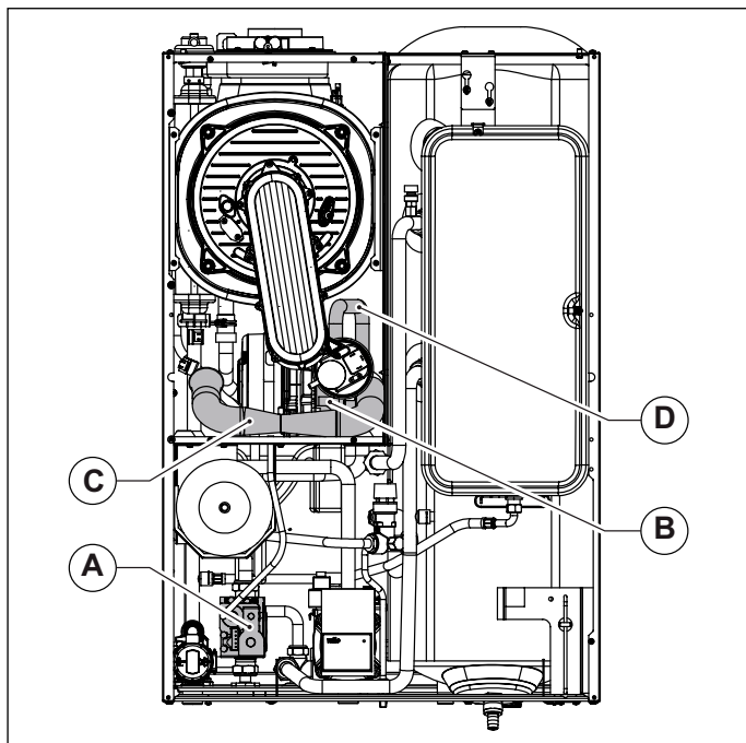
Fig. 26 Silenciador de aspiración
