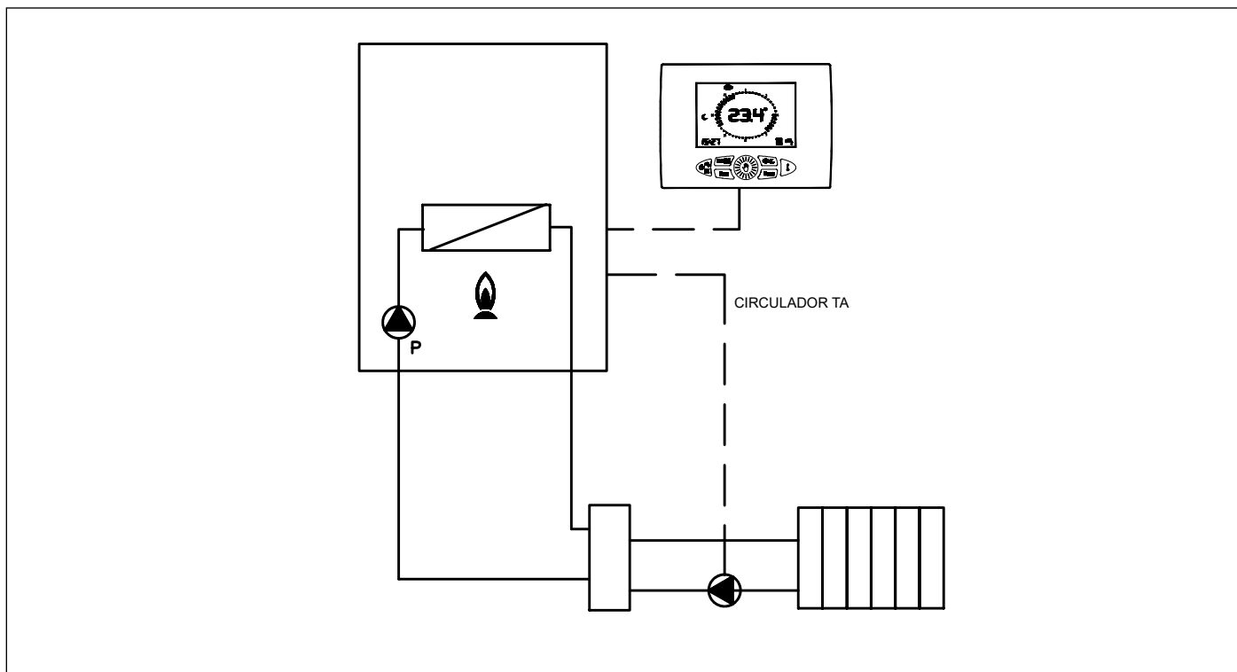
Fig. 23 Relé con pedido a distancia (P17=1)
