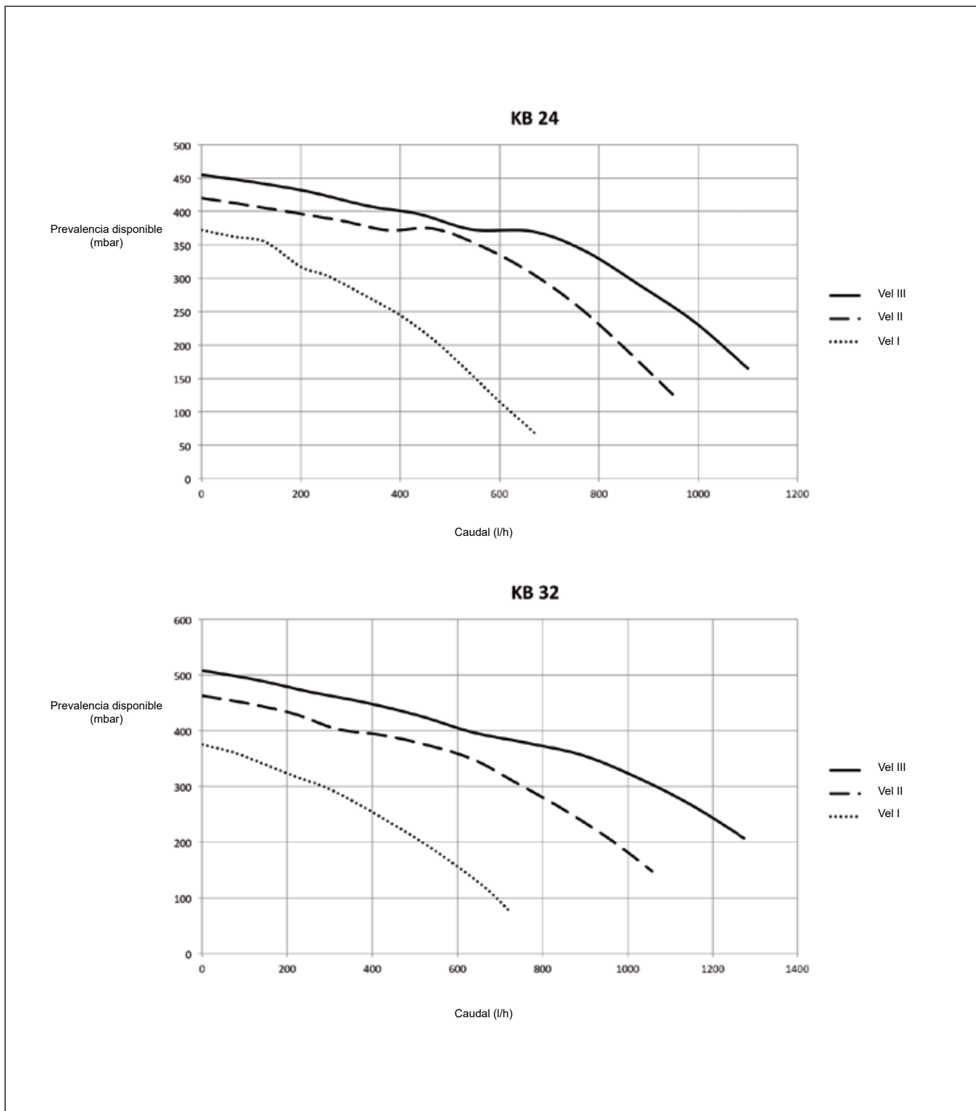
Fig. 17 Alturas residuales disponibles
