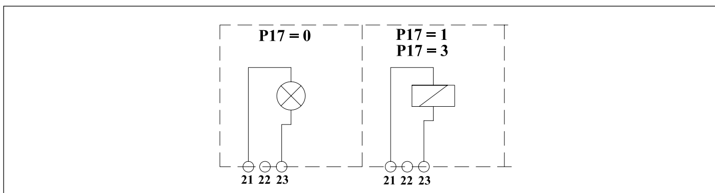
Fig. 20 Esquema de conexión relé multifunción
