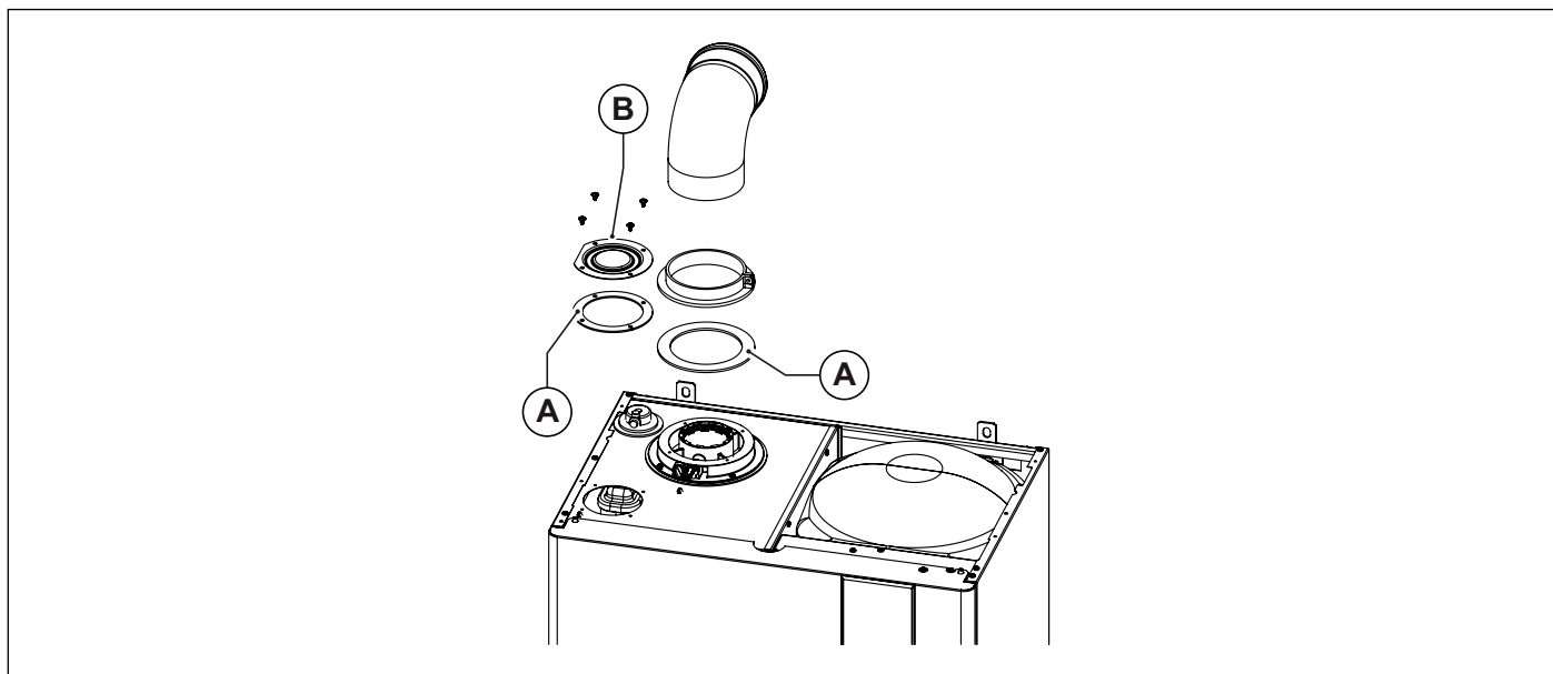
Fig. 9 Conductos coaxiales tipo C13 - C33
