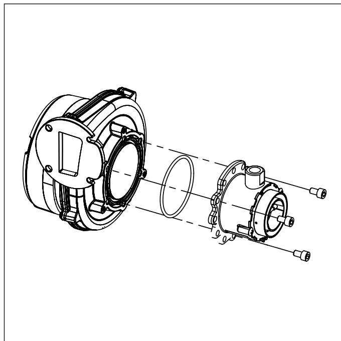
Fig. 27 Mezclador
