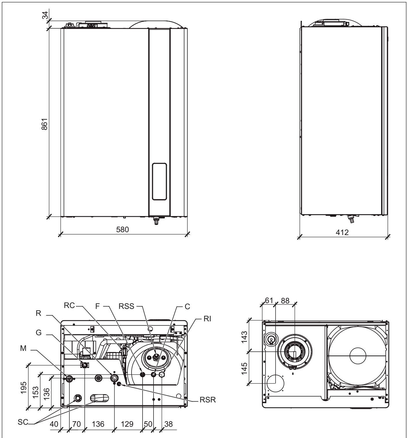
Fig. 3 Dimensiones
