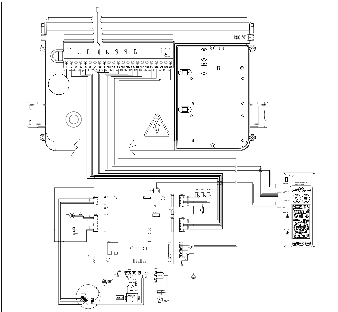
Fig. 18 Esquema eléctrico
